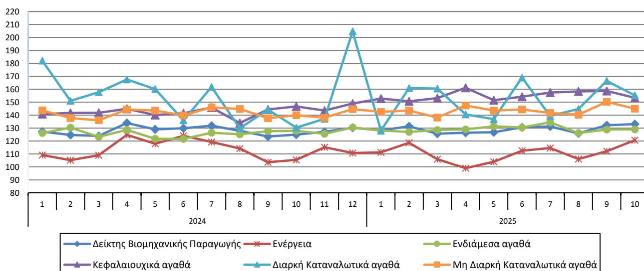
Γράφημα 6. Εξέλιξη του εποχικά διορθωμένου Γενικού Δείκτη Βιομηχανικής Παραγωγής και των Δεικτών Κύριων Ομάδων Βιομηχανικών Κλάδων, Ιανουάριος 2024 - Οκτώβριος 2025 (2015=100,0)
