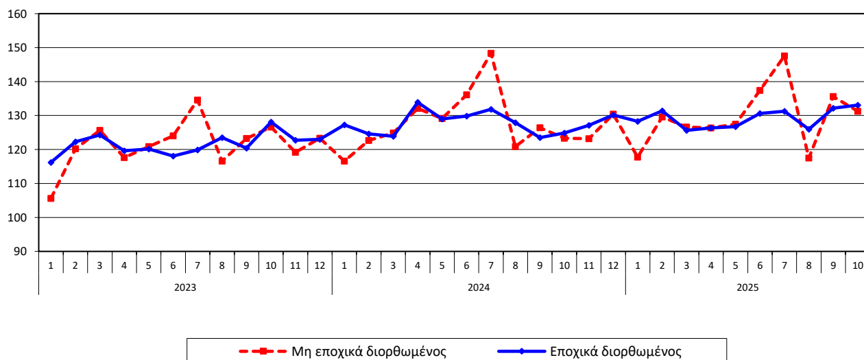
Γράφημα 4. Εξέλιξη Γενικού Δείκτη Βιομηχανικής Παραγωγής (2015=100,0)
